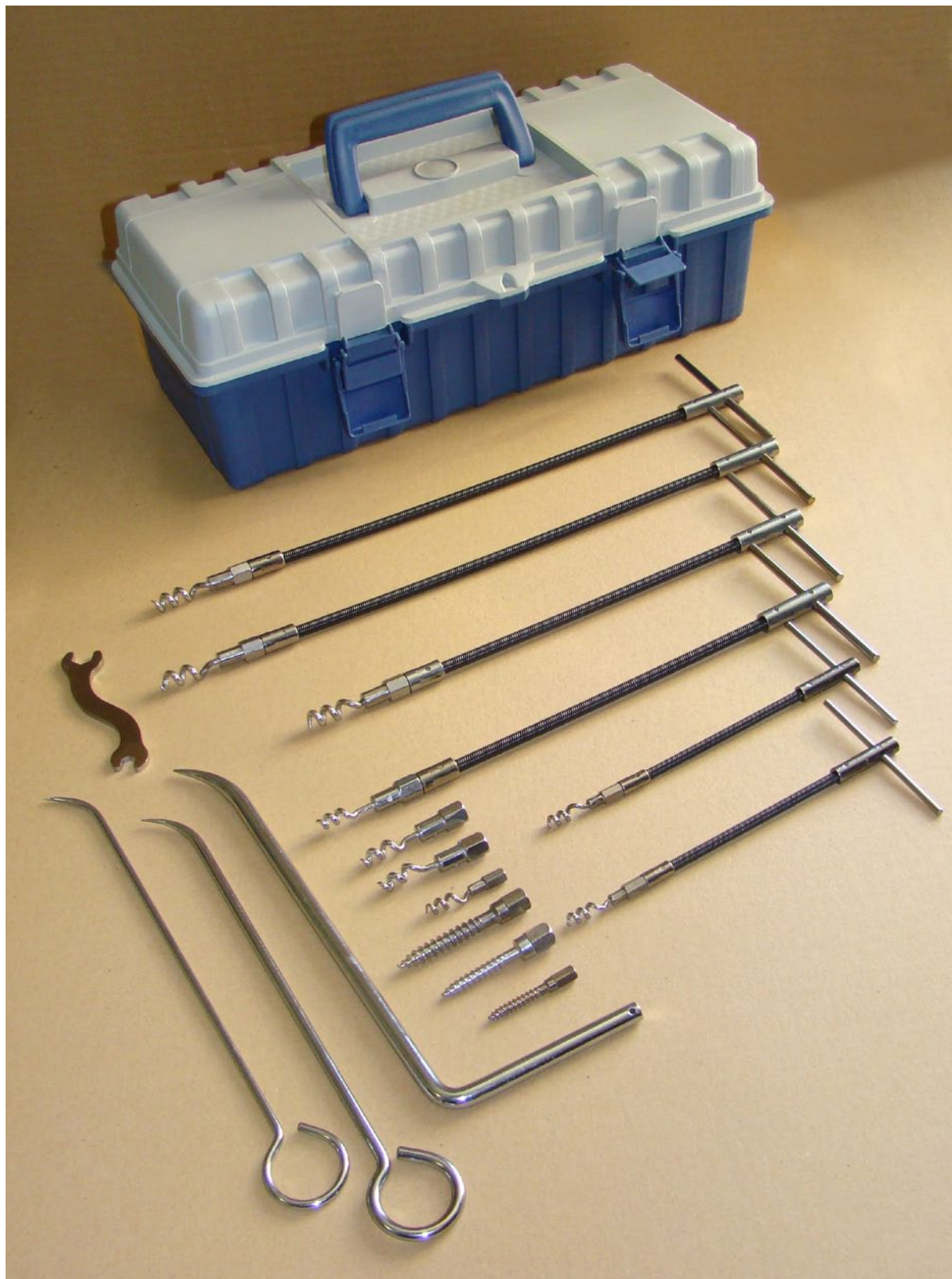
Sada vytahováků ucpávkových šňůr v přepravním boxu
